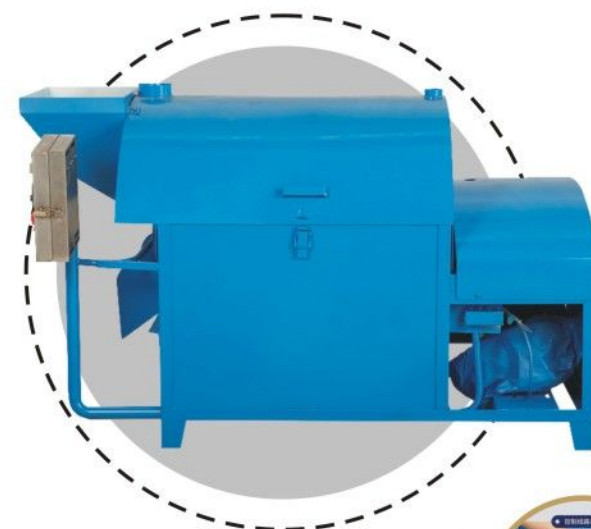
导电环式电加热滚筒炒货机 Electric nuts roasting machine
